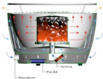
Il sistema ventilato di LotusGrill
